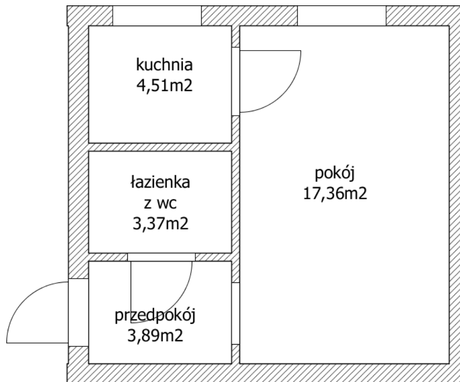
Struktura lokalu do remontu
